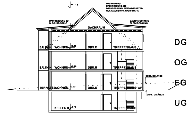
SCHNITT 3 - 3 (HAUS 3)
