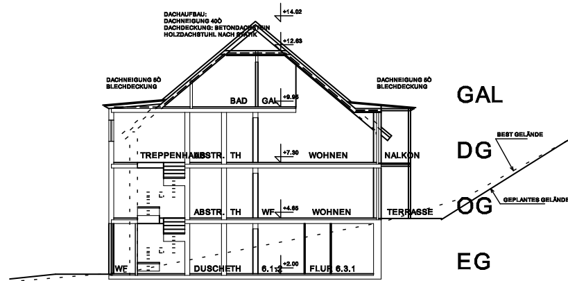
SCHNITT 4 - 4 (HAUS 4)
