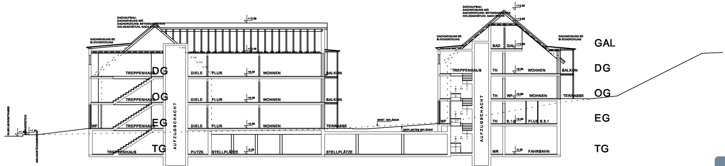
SCHNITT 1-1 (HAUS 1 + HAUS 6)
