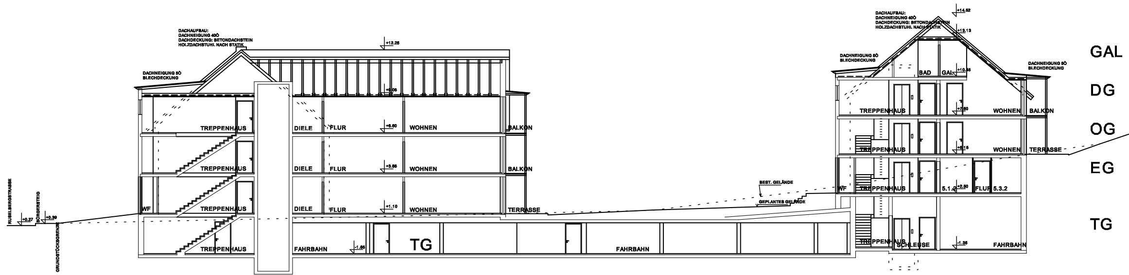
SCHNITT 2-2 (HAUS 2 + 5)
