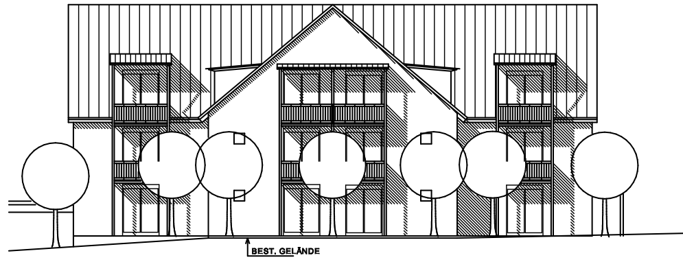
ANSICHT 1.3 (SÜDOSTEN)
