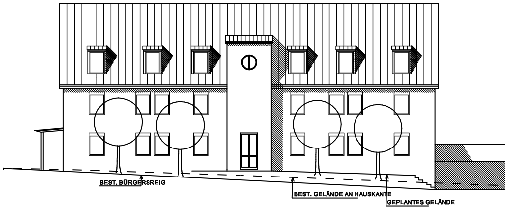
ANSICHT 1.1 (NORDWESTEN)
