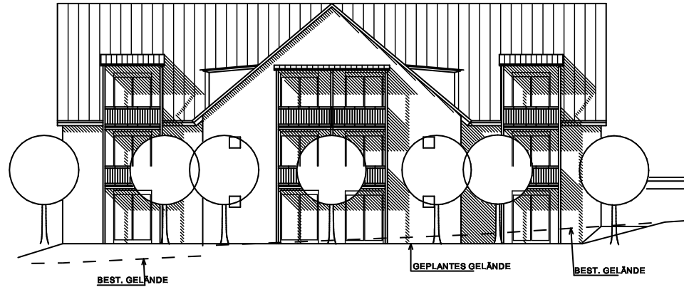
ANSICHT 2.3 (SÜDOSTEN)
