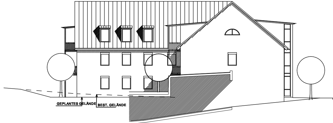
ANSICHT 2.4 (NORDOSTEN)
